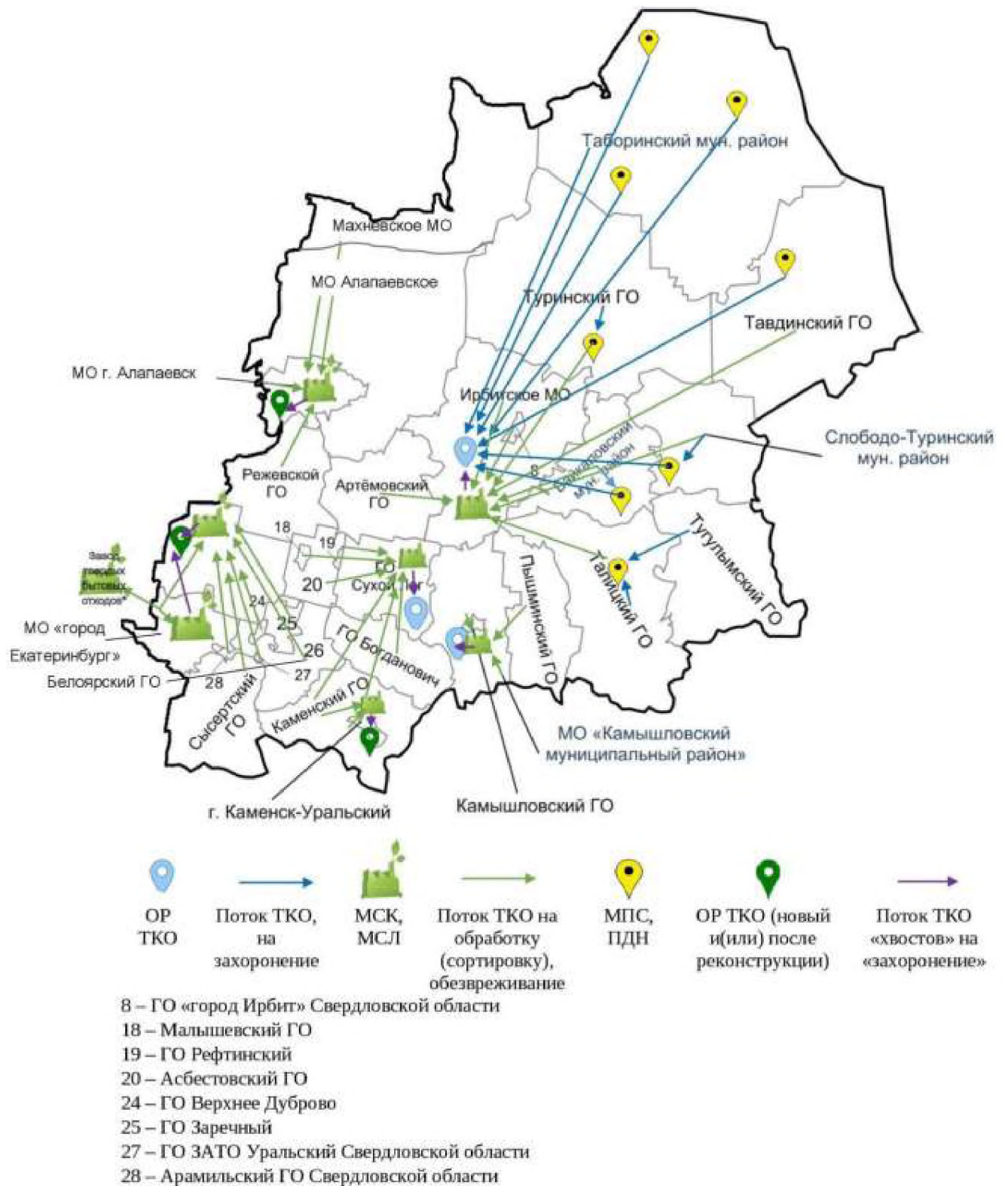
Рис. 14. Схема потоков TKO АПО-3 (IV этап) – 1 вариант
