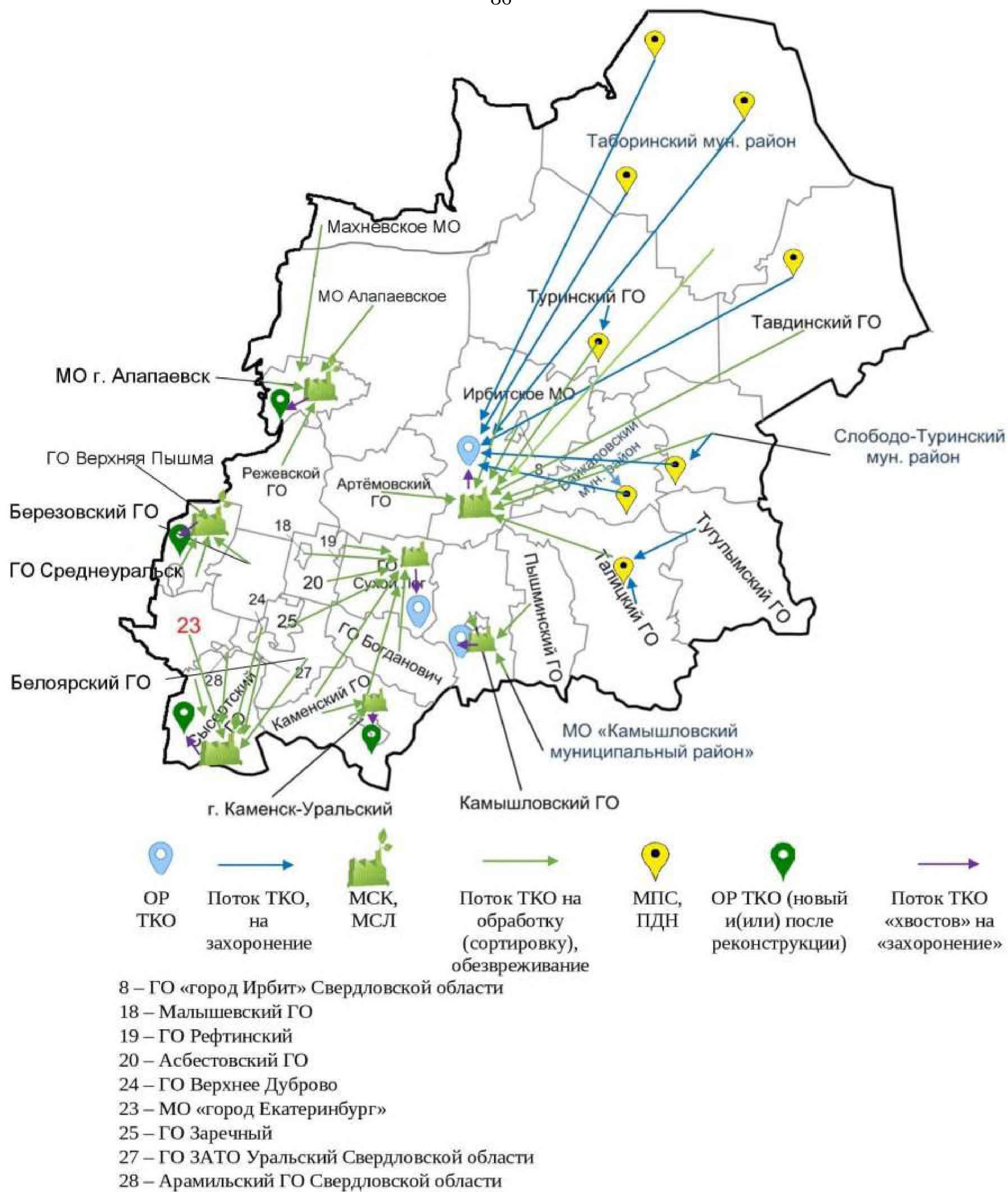
Рис. 11. Схема потоков ТКО АПО-3 (II этап) – 2 вариант
